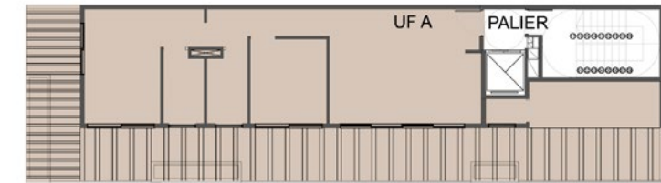
PLANTA TIPO 7
